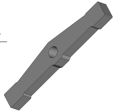
Rocker arm KPG-401-020-002
