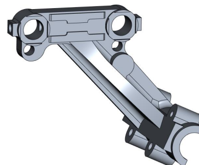
Корпус KPG-401-018-001
