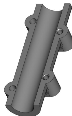
Крышка KPG-401-004-002
