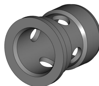
Втулка KPG-401-001-005
