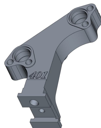
Корпус KPG-401-014-001
