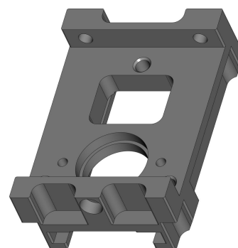
Плита KPG-401-009-002
