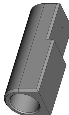
Держатель KPG-401-006-003
