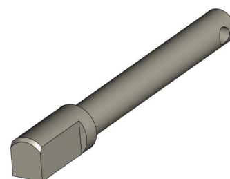
Фиксатор KPG-401-006-011
