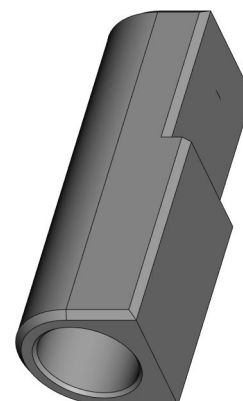
Holder KPG-401-006-003
