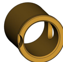
Bushing KPG-401-006-004
