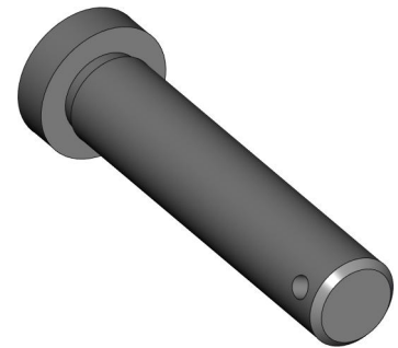
Finger KPG-401-004-010
