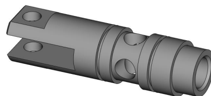
Шток головки KPG-401-003-003-001
