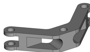
Rocker arm KPG-401-003-004
