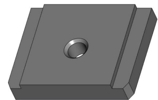
Сухарь KPG-401-001-007-001
