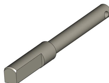
Фиксатор KPG-401-001-009
