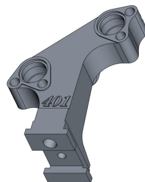
Корпус KPG-401-002-001
