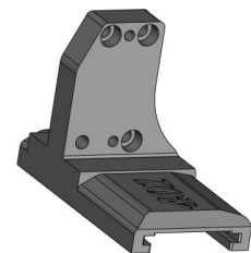
Кронштейн левый DGK-401-010-003
