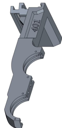
Стойка левая DGK-401-034-002
