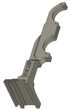
Стойка левая DGK-401-031-001
