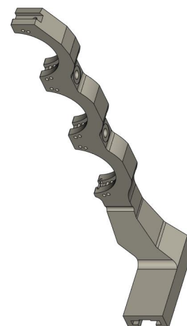
Стойка правая DGK-401-021-002
