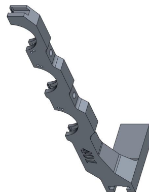
Стойка левая DGK-401-020-003
