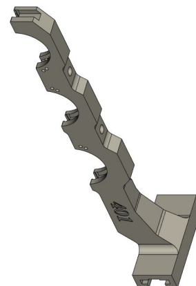
Стойка правая DGK-401-019-001
