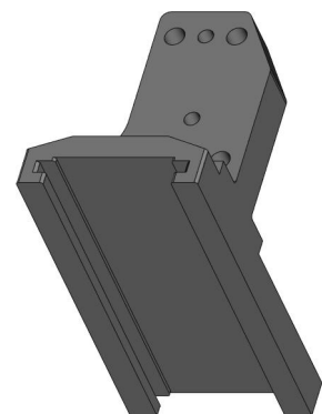
Фиксатор DGK-401-014-002
