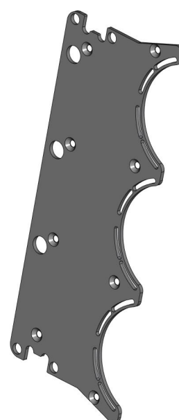
Плита DF-401-050-003-003
