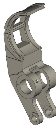
Рычаг нижний DF-401-043-001
