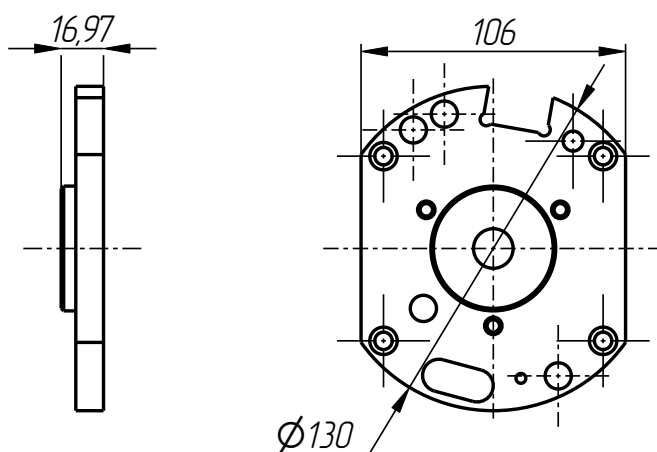
Cap assembly MPL-401-021-002
