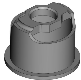
Стакан PPL-401-017-003
