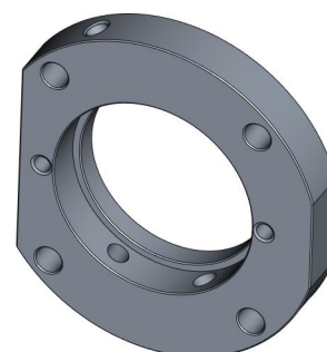
Фланец PPI-401-061-002
