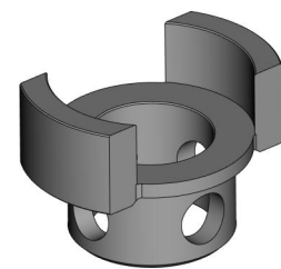
Стакан PPL-401-023-002
