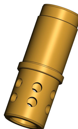
Гильза PPL-401-035-002
