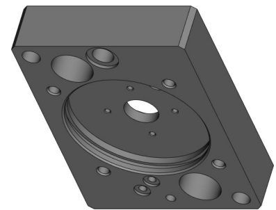
Крышка MPL-401-018-008-001
