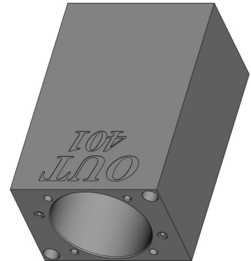
Корпус MPL-401-018-001
