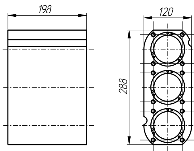
Корпус в сборе MPL-401-016-001
