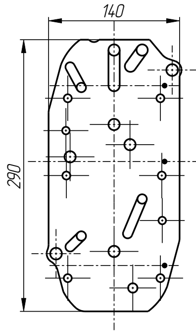
Плита в сборе MPL-401-015-007
