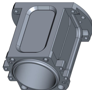
Цилиндр MPL-401-009-001-001
