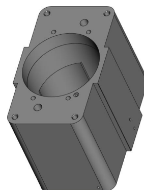
Мain body MPL-401-008-004-001
