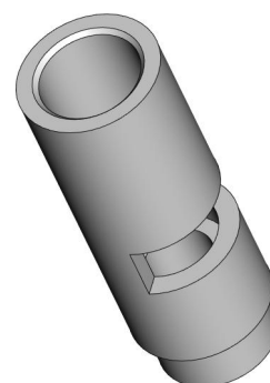
Держатель MPL-401-005-001-002
