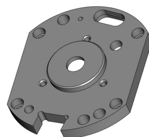
Крышка MPL-401-001-005-001
