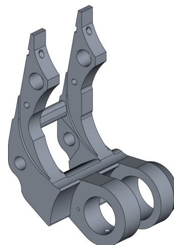
Рычаг верхний DF-401-036-002
