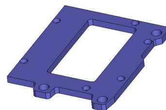
5. Bottom plate ELP-401-003
