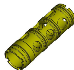
1. Корпус клапана KLO-401-005-001
