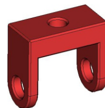
7. Скоба ПКБСТ-400-04-7
