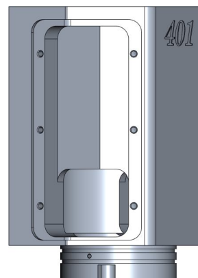
Цилиндр MPL-401-010-004-001
