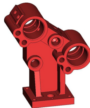
1. Корпус KDG-401-011-001
