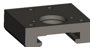
2. Плита монтажная kdg-401-009-002
