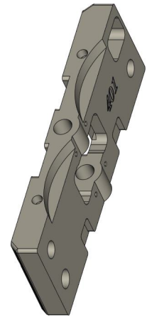
Плита правая DF-401-029-001-001
