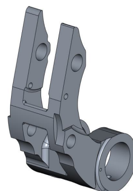
Рычаг верхний DF-401-026-002
