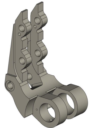
Рычаг нижний DF-401-023-001
