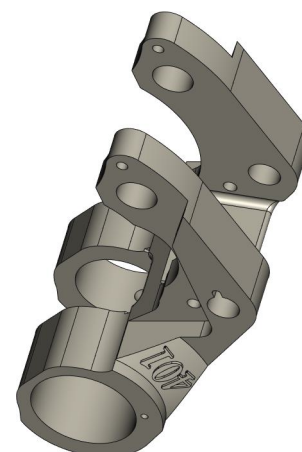
Рычаг нижний DF-401-007-001
