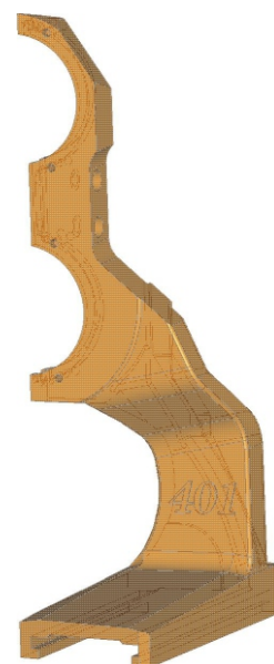
1. Держатель правый DGK-401-004-001
