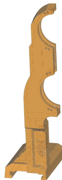
1. DGK-401-003-001 Держатель правый
