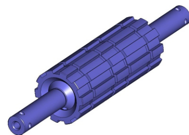
1. Вал шлицевой MT-401-001-001
