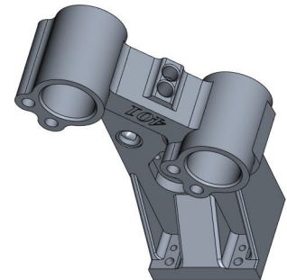
Кронш KDG-401-001-001
