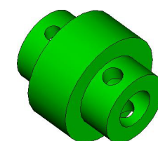
8. Gear MKO-401-002-004
